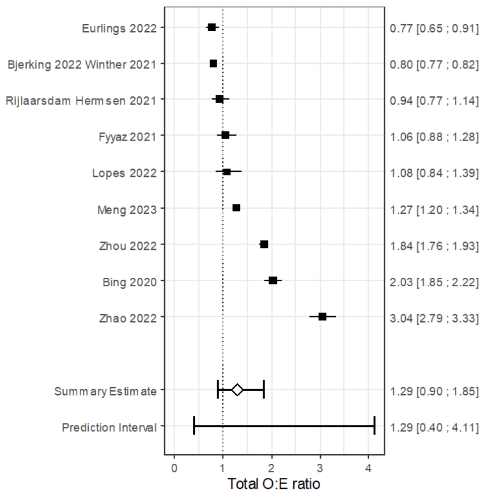
Figur 5. Metaanalys av O:E-kvot (Observed/Expected). Punktestimat med tillhörande konfidensintervall representeras av romben. Prediktionsintervallet indikerar ett spann där kommande studier kan hamna.
