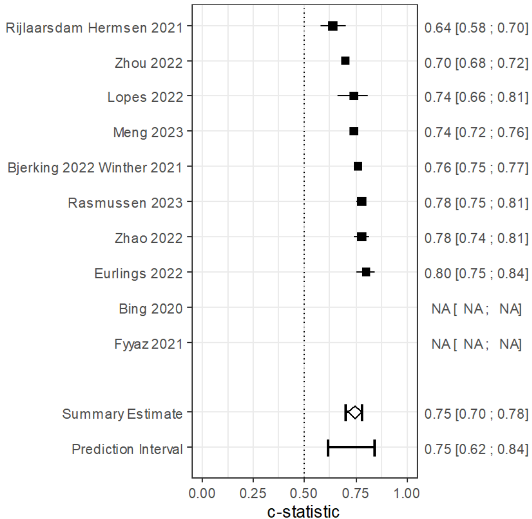
Figur 4. Metaanalys av AUC. Punktestimat med tillhörande konfidensintervall representeras av romben. Prediktionsintervallet indikerar ett spann där kommande studier kan hamna. Prediktionsintervall blir vanligtvis brett om det finns färre än 10 studier.
